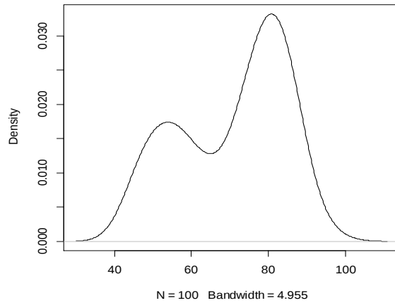
Fig. 5 nrd0 –Default Bandwidth
